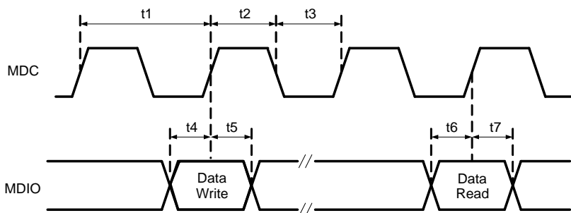
Figure 22. SMI (MDC/MDIO) Timing
